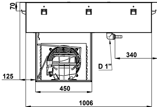
Zij aanzicht
